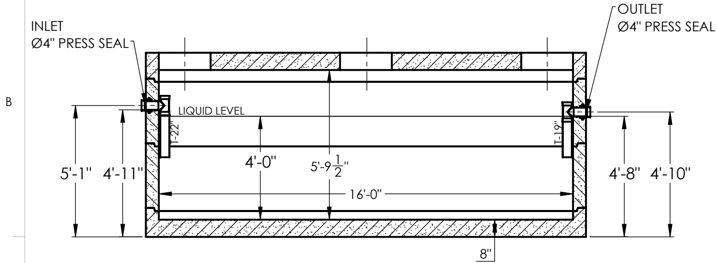
SECTION A-A
